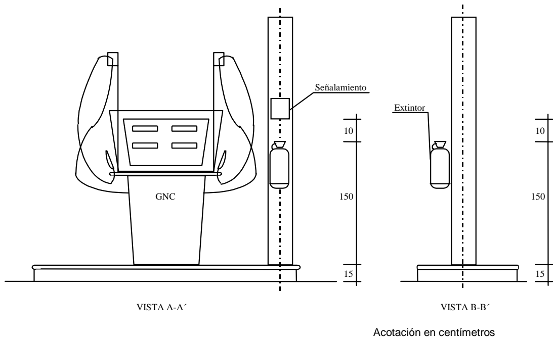
Fig 3.- Localización de los surtidores sobre un módulo de abastecimiento distancias mínimas requeridas en estaciones públicas de servicio
