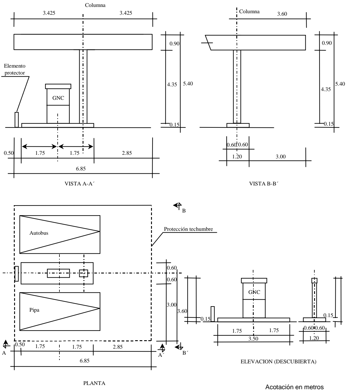
Fig 1.- Techumbre, módulo de abastecimiento sencillo y distancias mínimas requeridas para estaciones de servicio de GNC.
