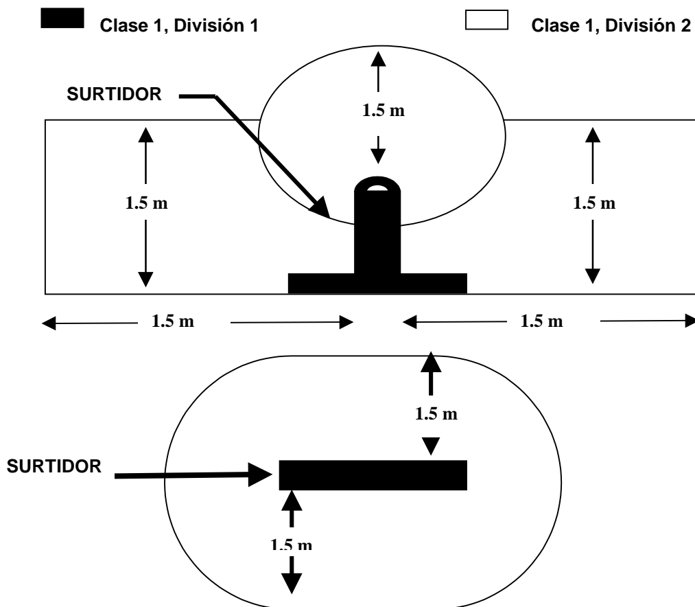
Fig. 6.- Distancias de seguridad de los surtidores
